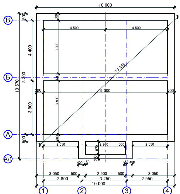
План фундамента
