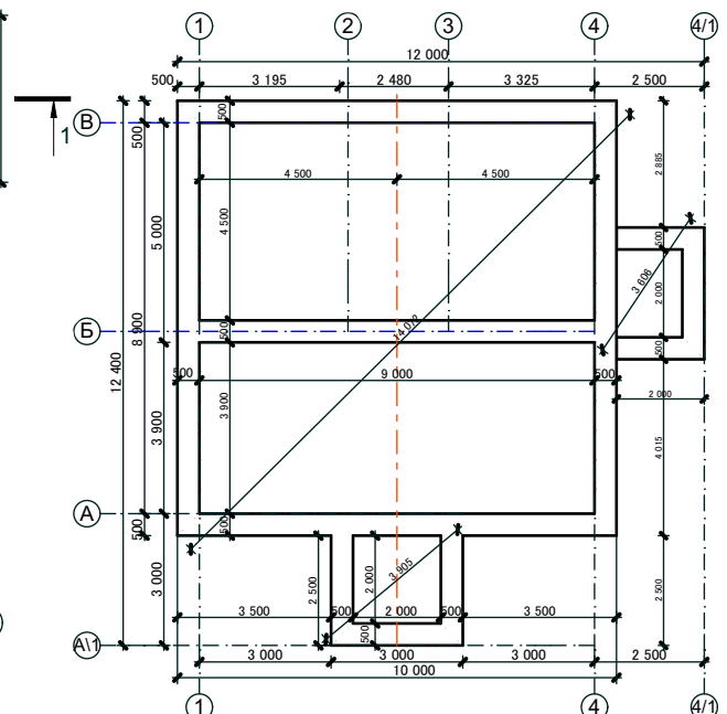
План фундамента
