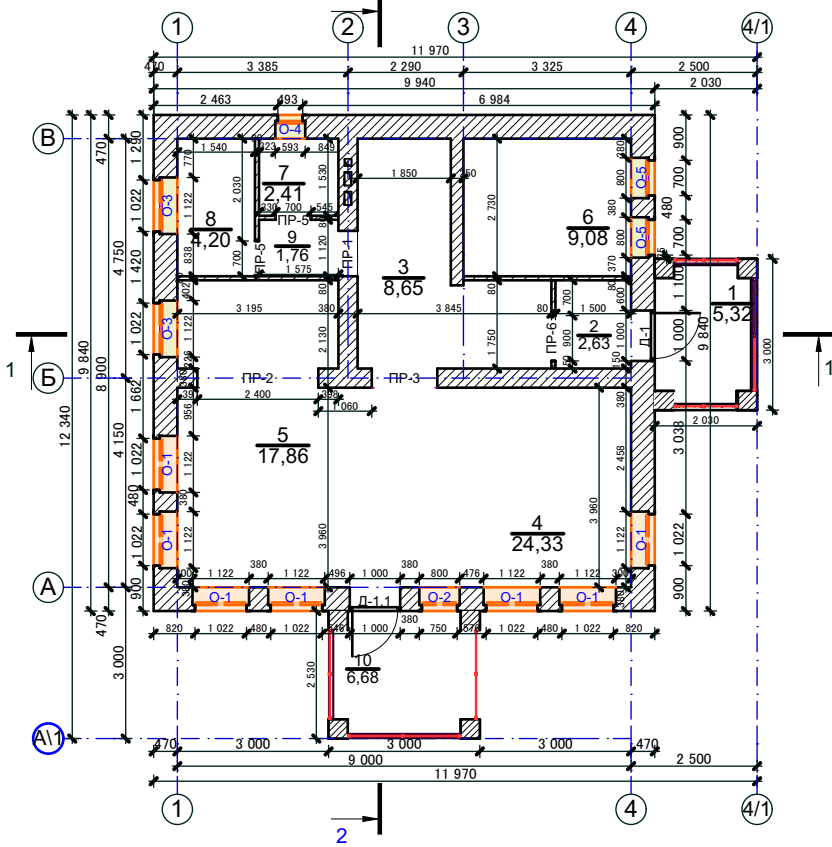
План 1-ого этажа
