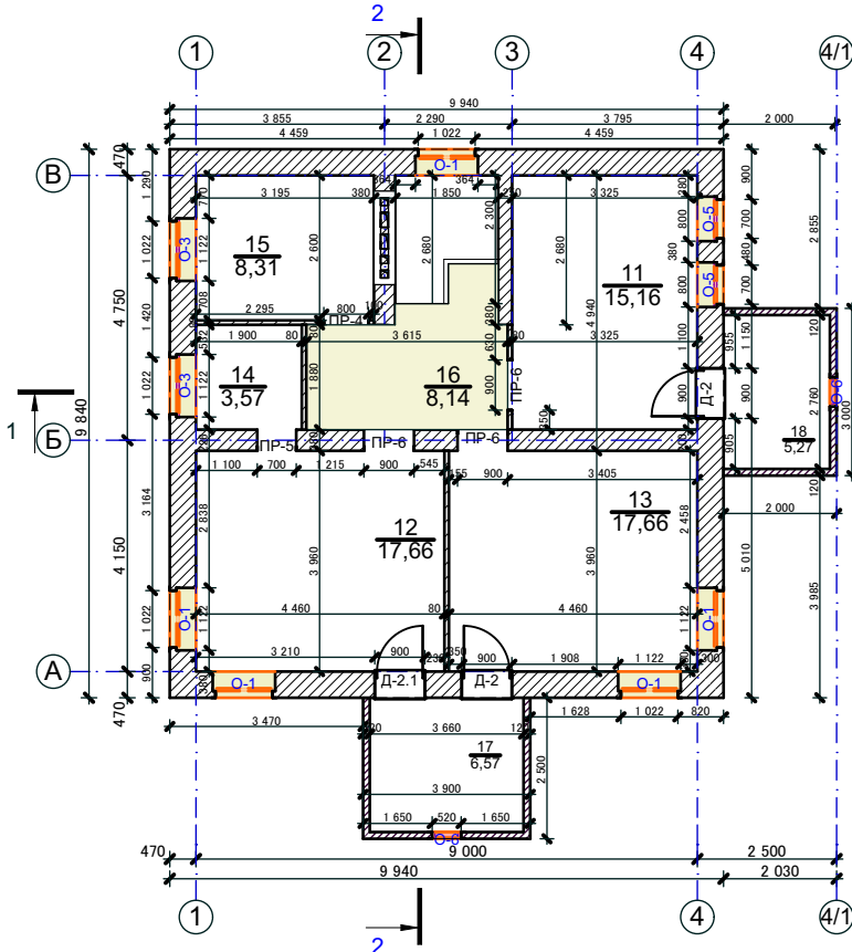
План 2-ого этажа
