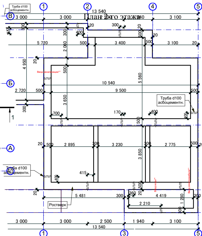
План фундаментов
